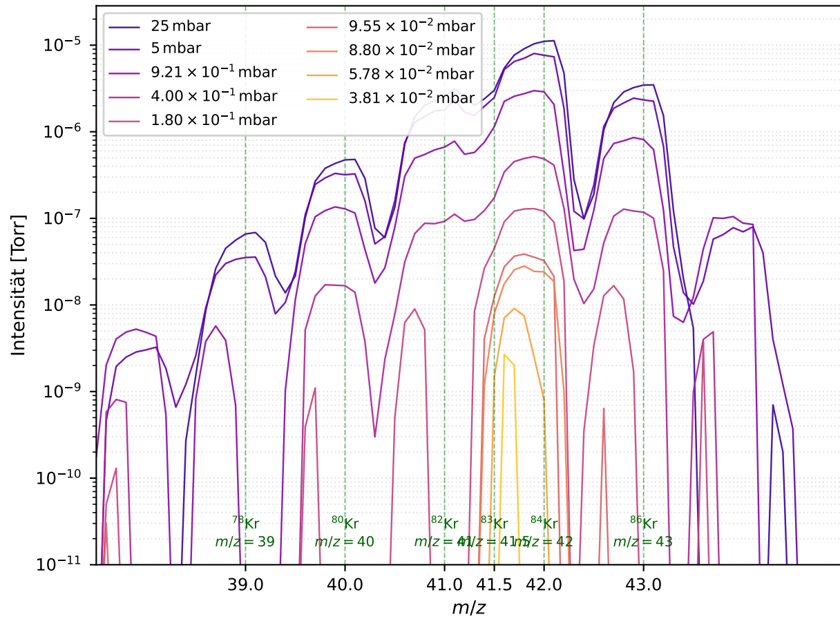
(b) \text{Kr}^{2+} — doppelt ionisiert ( m/z = A/2 )
