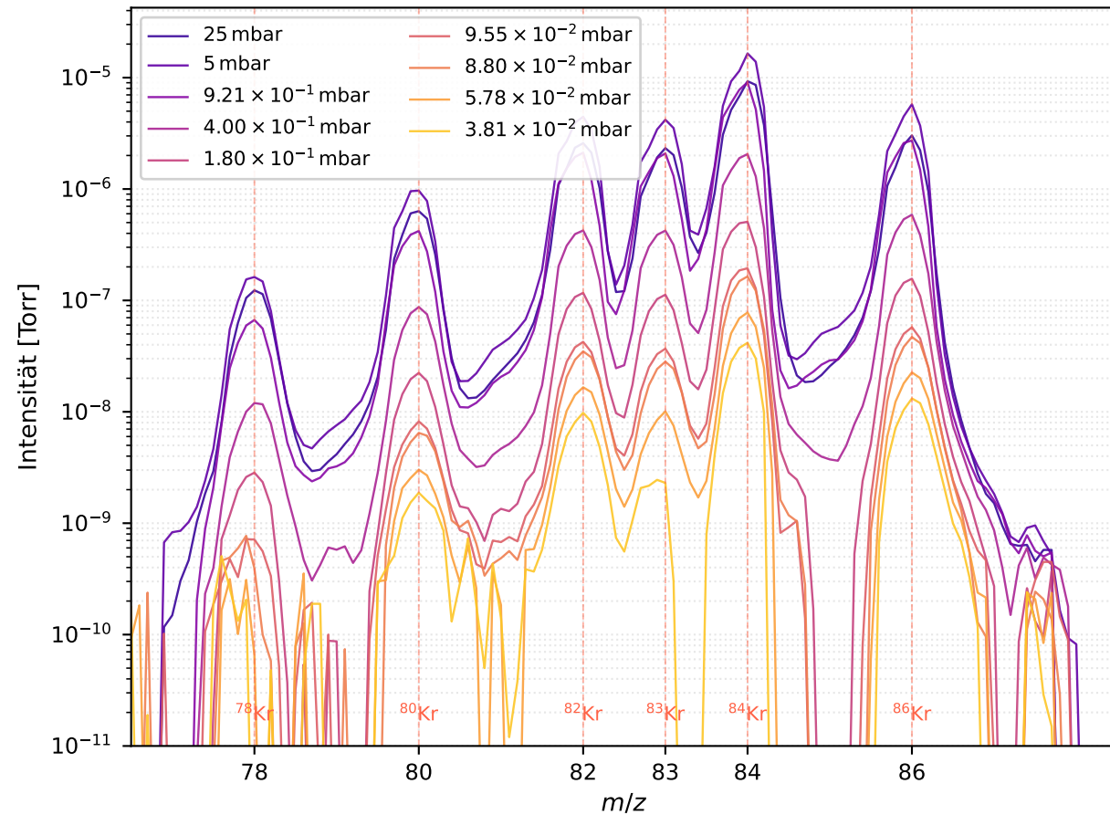
(a) \text{Kr}^+ — einfach ionisiert ( m/z = A )
